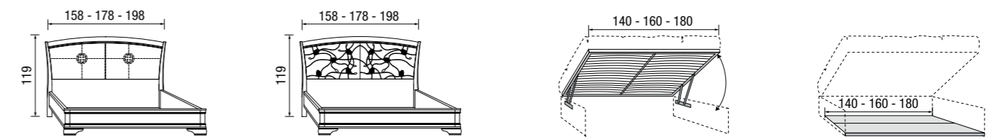
P. - D. - Г. 221 cm L. 158 * 71CI33LT L. 178 * 71CI34LT L. 198 * 71CI35LT P. - D. - Г. 221 cm L. 158 ** 71B033LT L. 178 ** 71B034LT L. 198 ** 71B035LT P. - D. - Г. 200 cm L. 140 71FE03RT L. 160 5B070211 L. 180 5B070212 P. - D. - Г. 200 cm L. 140 * 71CI03PN ** 71B003PN L. 160 * 71CI04PN ** 71B004PN L. 180 * 71CI05PN ** 71B005PN
