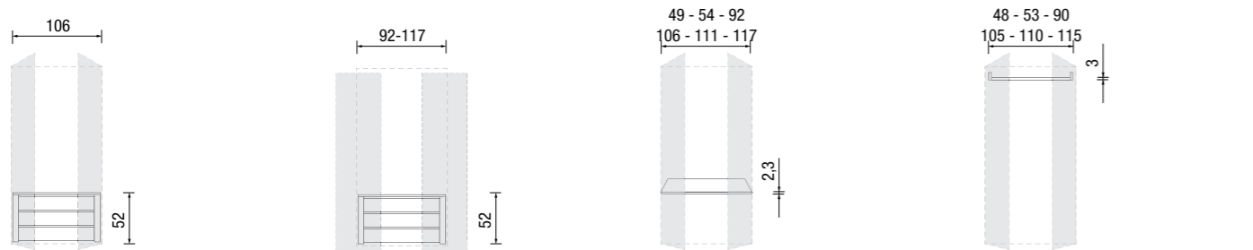
P. - D. - Г. 52 cm * 71CI01CE ** 71B001CE P. - D. - Г. 52 cm L. 92 * 71CI02CE ** 71B002CE L. 117 * 71CI03CE ** 71B003CE P. - D. - Г. 52 cm L. 49 * 71CI15CL ** 71B015CL L. 54 * 71CI13CL ** 71B013CL L. 92 * 71CI17CL ** 71B017CL L. 106 * 71CI14CL ** 71B014CL L. 111 * 71CI12CL ** 71B012CL L. 117 * 71CI18CL ** 71B018CL P. - D. - Г. 1,5 cm L. 110 71KT12FE L. 53 71KT13FE L. 105 71KT14FE L. 48 71KT15FE L. 90 71KT17FE L. 115 71KT18FE
